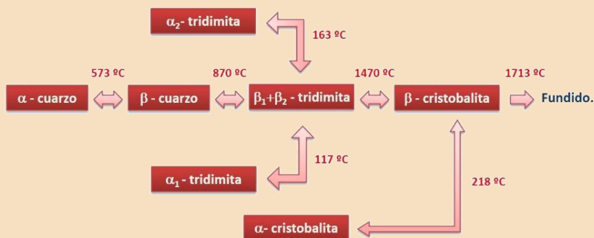
Figura 3. Transformaciones alotrópicas de la sílice. Imagen: Rafa Galindo.
